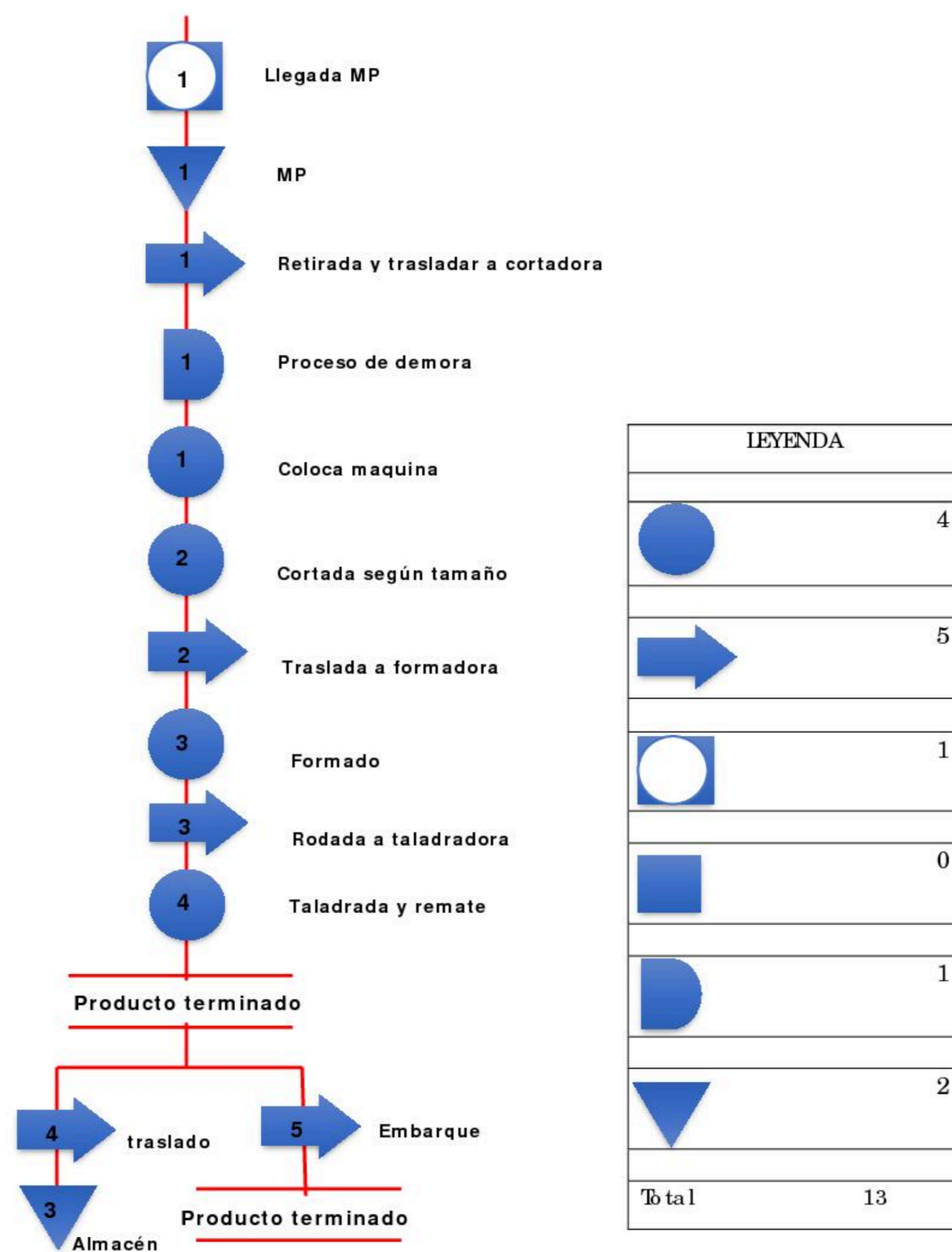
Figura 10: Ejemplo de Diagrama de Análisis del Proceso - DAP - Tubería Corrugada Para Alcantarillado. Tomada de Introducción a la Ingeniería Industrial, por A. Camacho, 2008, p. 66.
